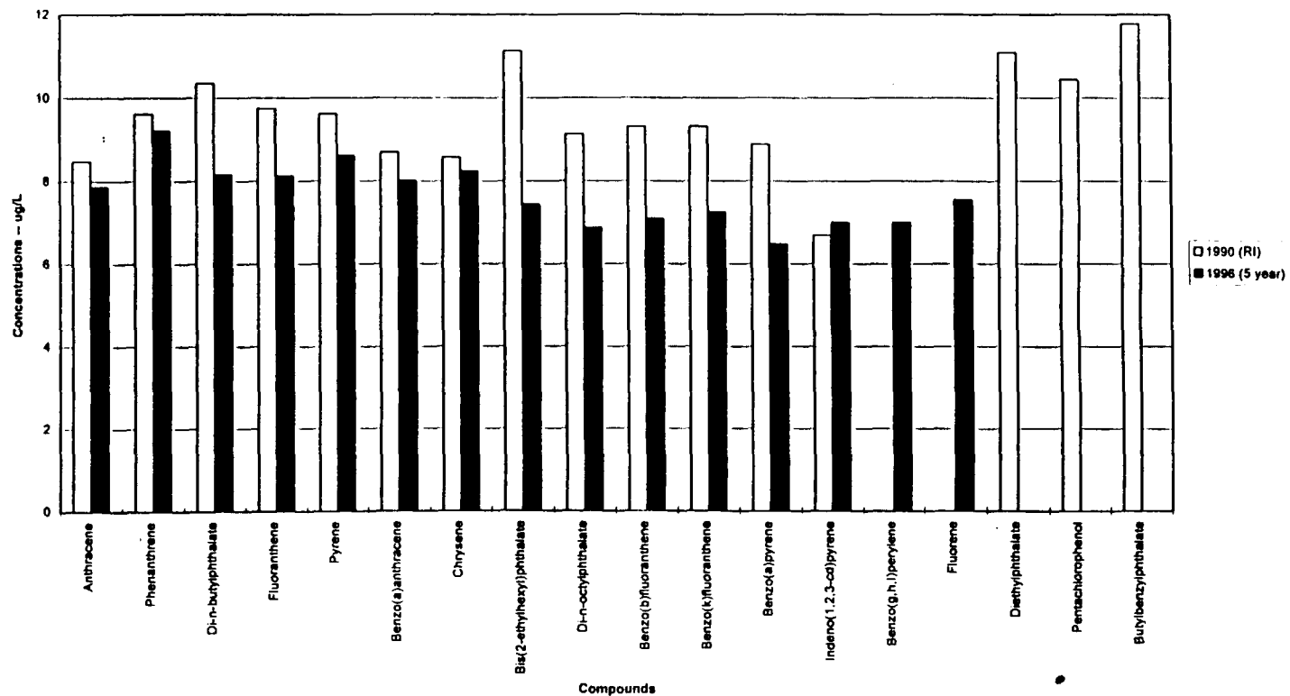
SVOC Trend In Quarry Sediments
