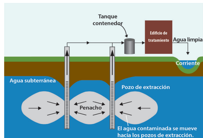
Ejemplo de un sistema de bombeo y tratamiento con dos pozos de extracción.
