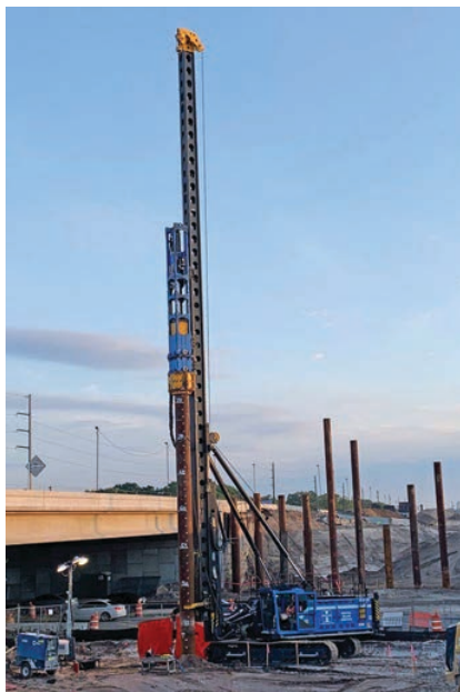
Leader rig
